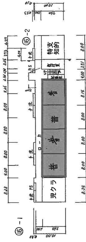
普通教室棟 1 階
